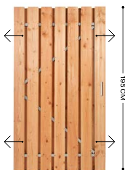
147303 geschaafd, universeel, 195 x 100 cm.
