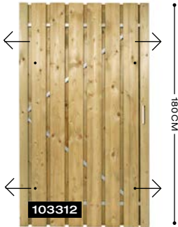
Vuren stalen frame deur, universeel, 180 x 100 cm.
